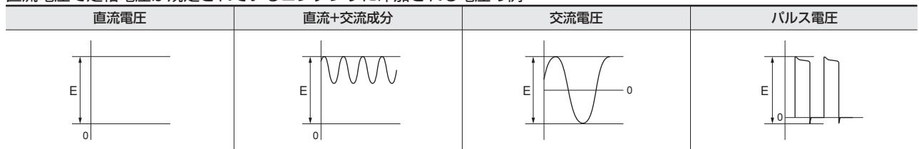
直流電圧で定格電圧が規定されているコンデンサに印加される電圧の例
